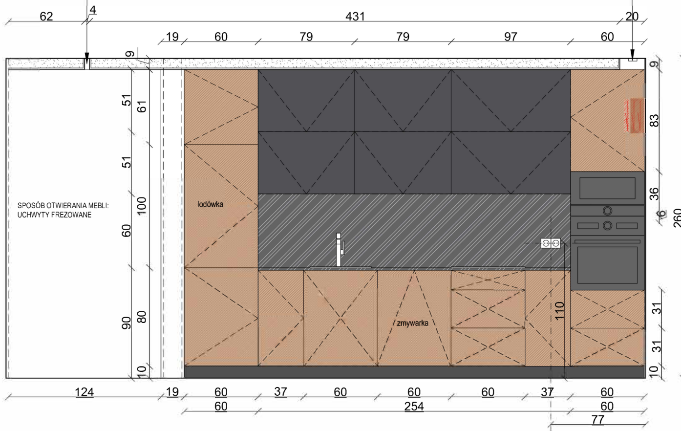
WIDOK K.1
