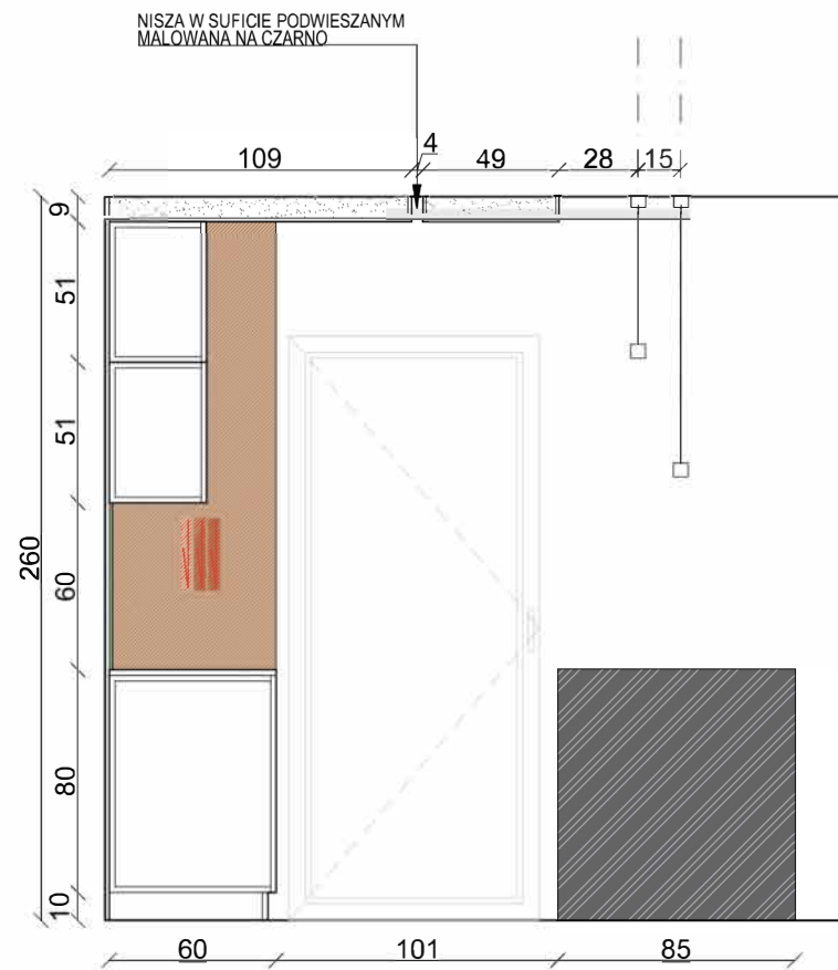
WIDOK K.5
