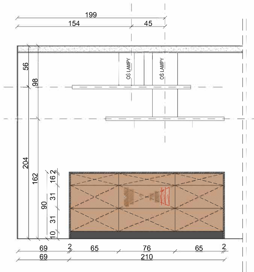
WIDOKK.3
